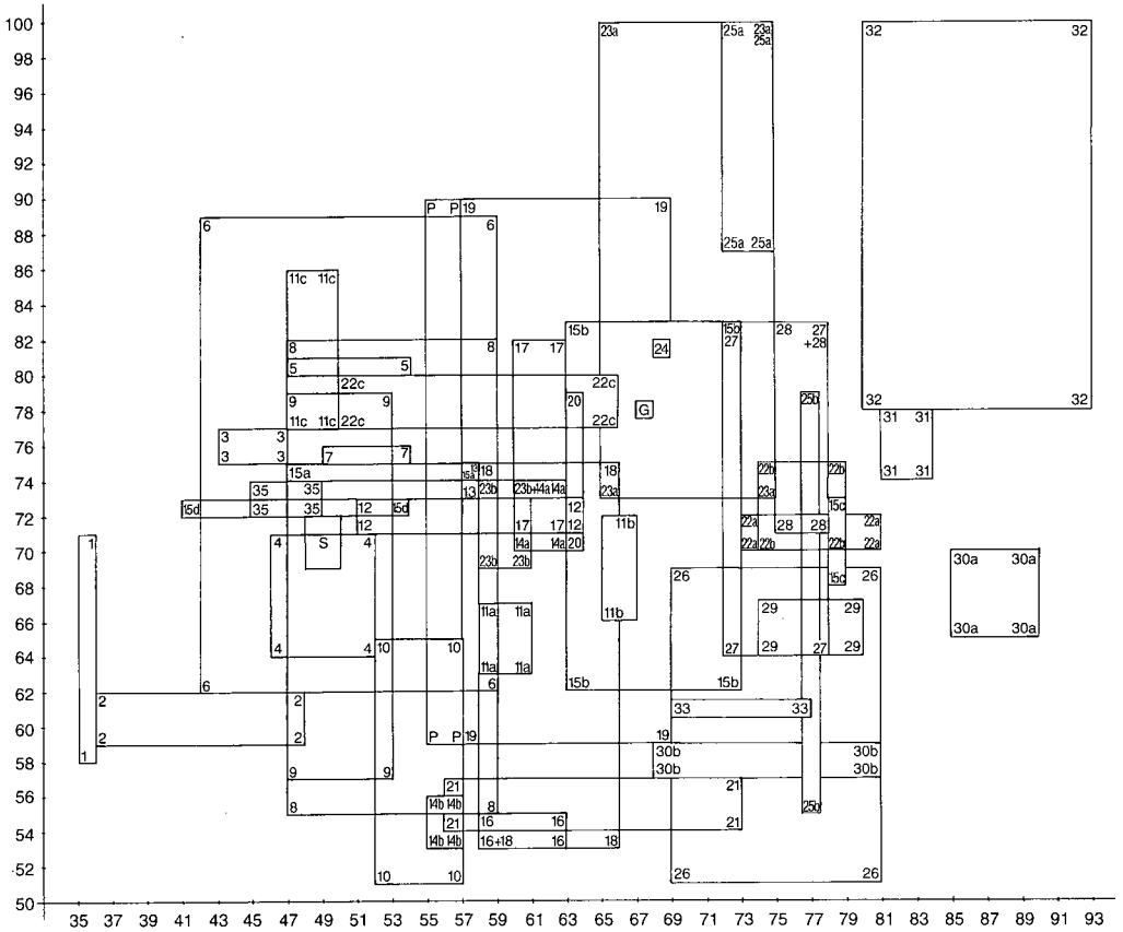
Abb. 3: Streuung der Breiten (= BI)- und Längen (= LI)-Indizes von Spleniale-Zähne der Gattung Coelodus .– vgl. Appendix 2.
