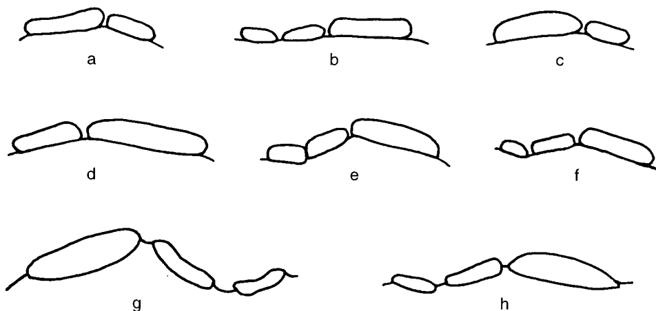
Abb. 2: Spleniale-Profile von Coelodus in neutraler (= horizontaler) Lage, natürl. Größe.
