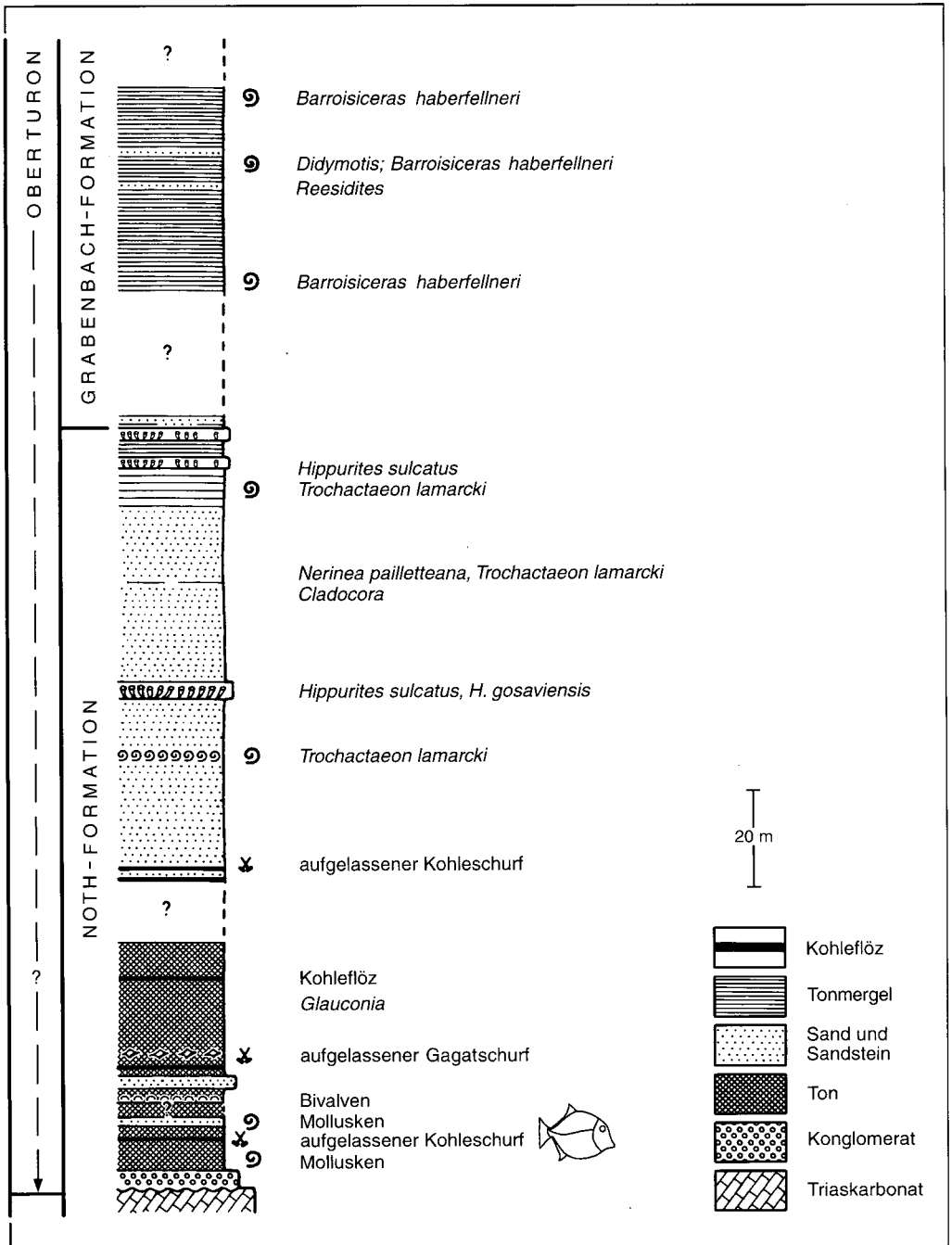
Abb. 1b: Vermessenes und kombiniertes Profil durch die Transgressionsserie der Gosau-Gruppe von Gams bei Hieflau. Nach SUMMESBERGER & KENNEDY 1996 und einer unveröffentlichten Aufnahme von SUMMESBERGER & HÖCK-DAXNER, verändert nach SIEGL-FARKÁS & WAGREICH (im Druck). – Das Fischsymbol gibt die Fundposition des Fischkiefers im Profil an.
