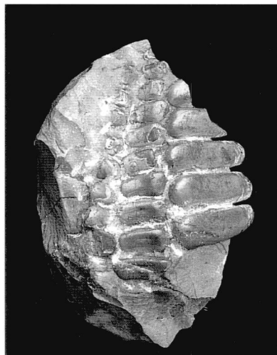
Abb. 9: Coelodus saturnus HECKEL, 1854; Bezahnungsreste des Spleniale dext., des Vomer, des Prämaxillare dext. und des Dentale dext. et sin. sowie Fragment des ? Angulare dext., Seitenansicht; Senonien; Prapatnica bei Trogir, Dalmatien, Kroatien.– HPM 9222.– natürl. Größe.
