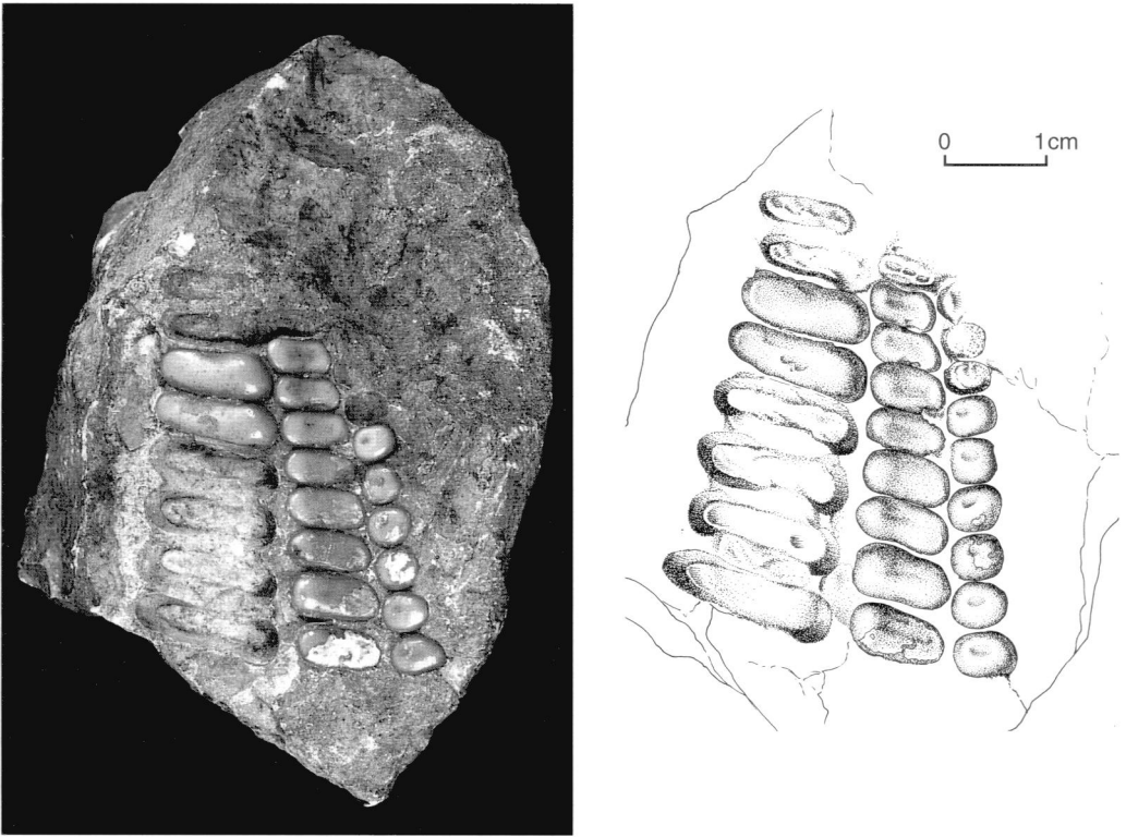
Abb. 12a+b: Coelodus cf. saturnus HECKEL, 1854; Spleniale dext. (Fragment), Aufsicht; Turonien; Starač, Insel Hvar, Kroatien.— HPM-ohne Nummer.— natürl. Größe.
