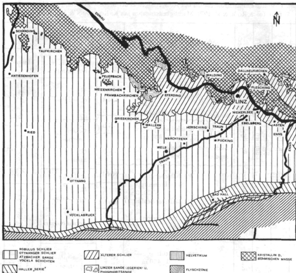
Abb. 2: Abgedeckte geologische Karte der Molassezone in Oberösterreich (nach BRAUMÜLLER 1961, etwas abgeändert) Maßstab 1 : 600.000.
