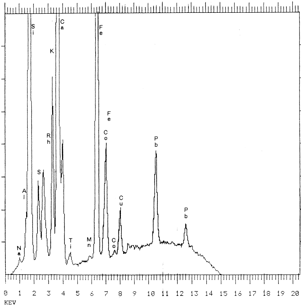
Abb. 7: Spektren der Elemente (blau) (DI G. HALMETSCHLAGER, Atominstitut Wien).
