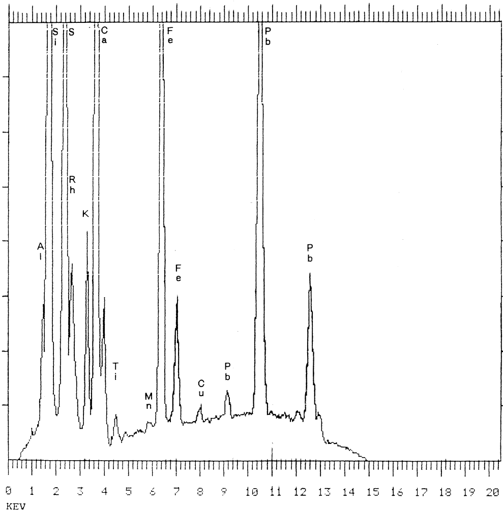
Abb. 5: Spektren der Elemente (gelb) (DI G. HALMETSCHLAGER, Atominstitut Wien).
