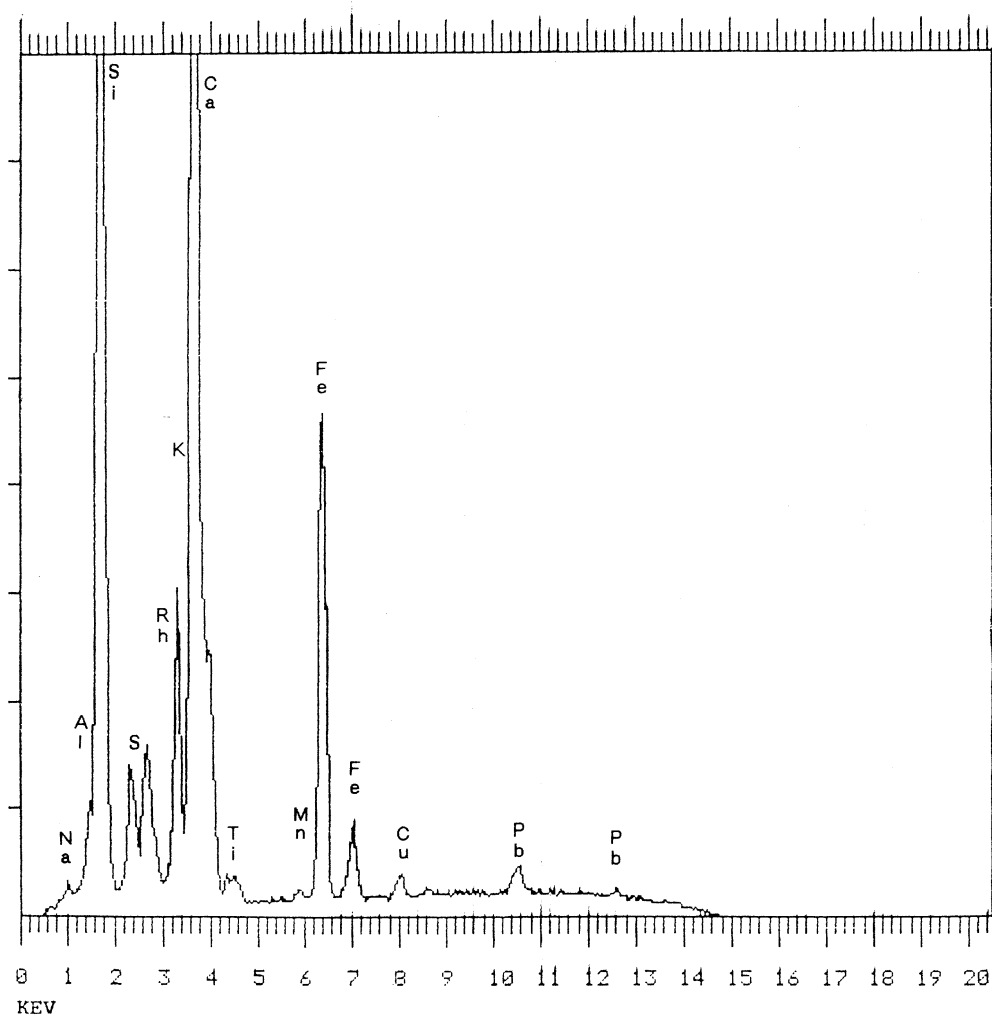
Abb. 6: Spektren der Elemente (weiß) (DI G. HALMETSCHLAGER, Atominstitut Wien).
