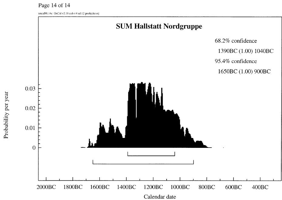
Abb. 2: Gruppenkalibration der Nordgruppe.
