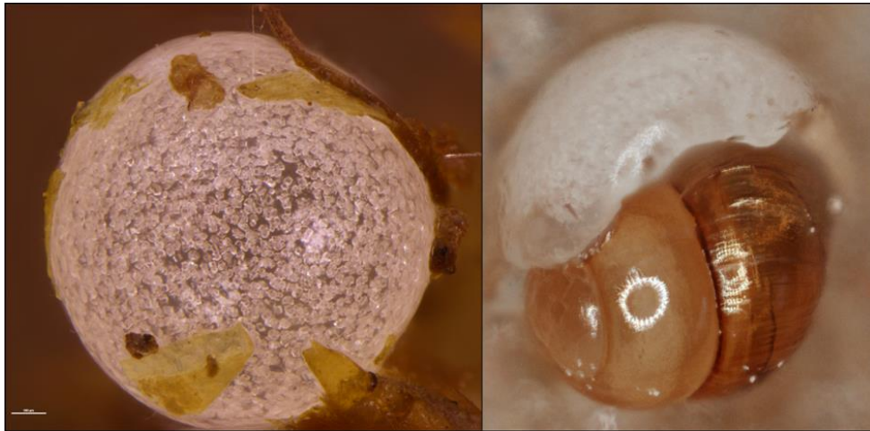
Abbildung 6. Clausilia dubia : Ei (links); O. Macek CC BY SA; schlüpfende Schnecke (rechts); © K. Jaksch
