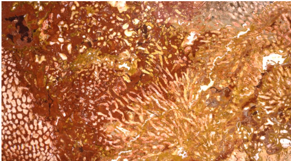
Abbildung 7. Polierte Platte mit Korallenstöcken eines Trias-Riffes. Adnet, Salzburg, 205 Millionen Jahre alt; © M. Harzhauser
